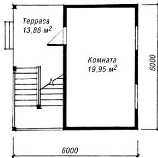
план первого этажа
