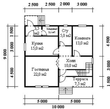
ПЛАН 1-ГО ЭТАЖА
