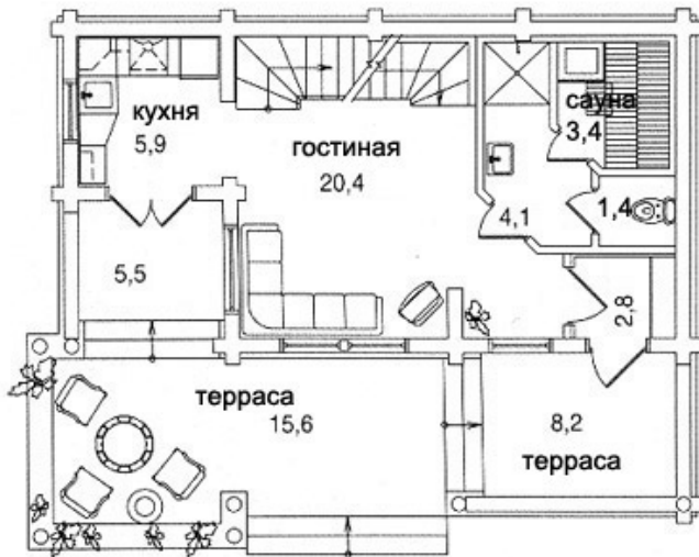
План 1 этажа
