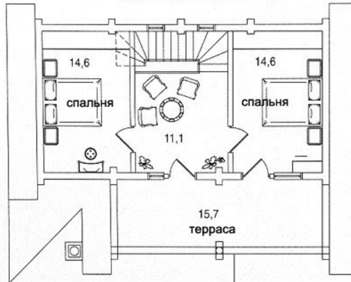
План 2 этажа
