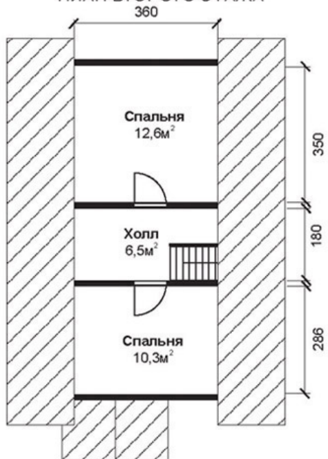
ПЛАН ВТОРОГО ЭТАЖА
