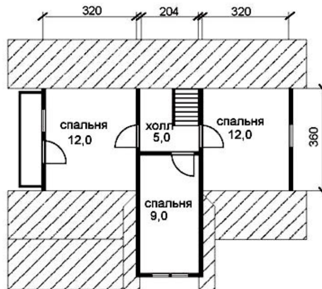
План 2 этажа
