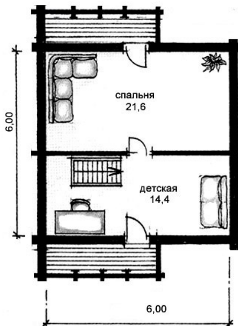
План 2 этажа
