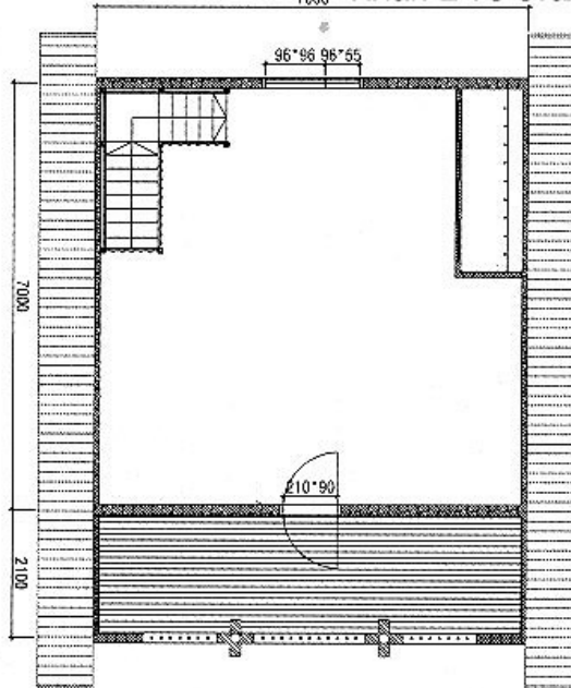
План 2-го этажа
