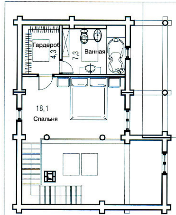
План 2 этажа
