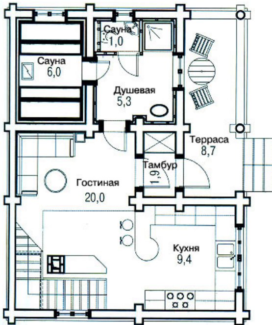
План 1 этажа
