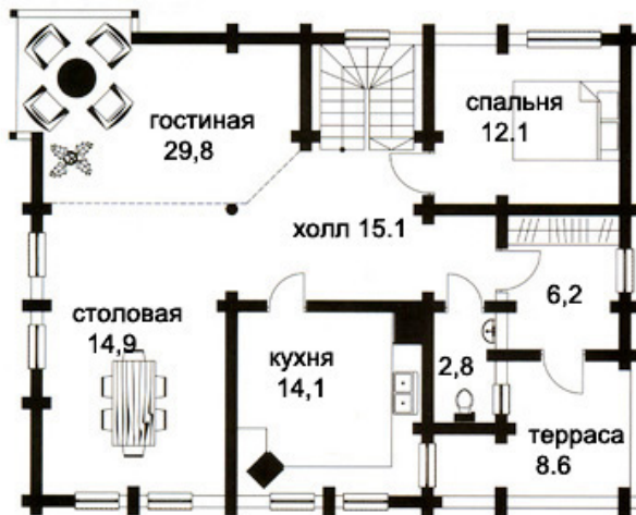
План 1 этажа
