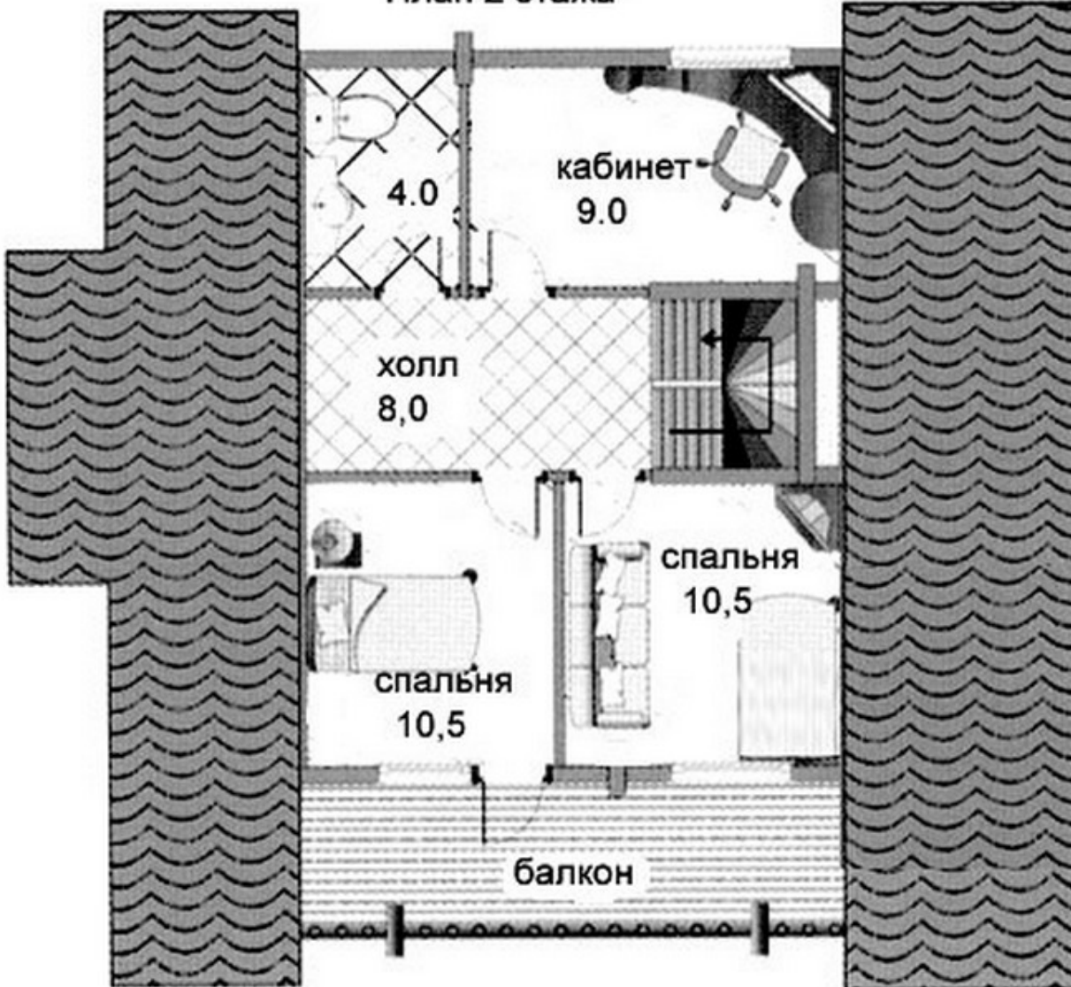
План 2 этажа
