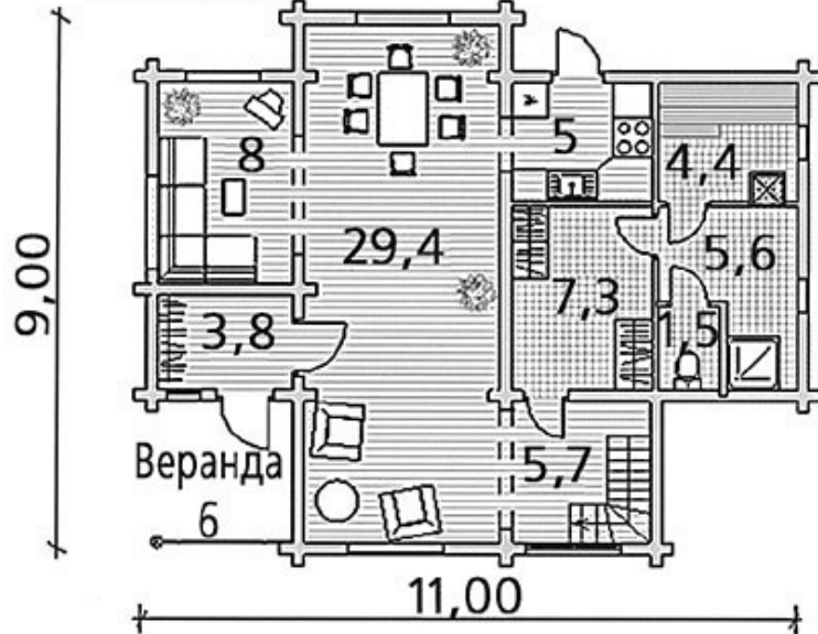
План 1 этажа
