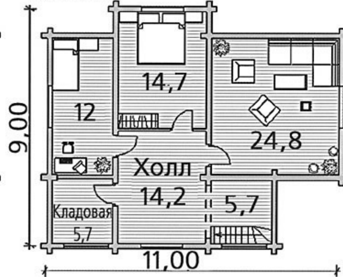
План 2 этажа
