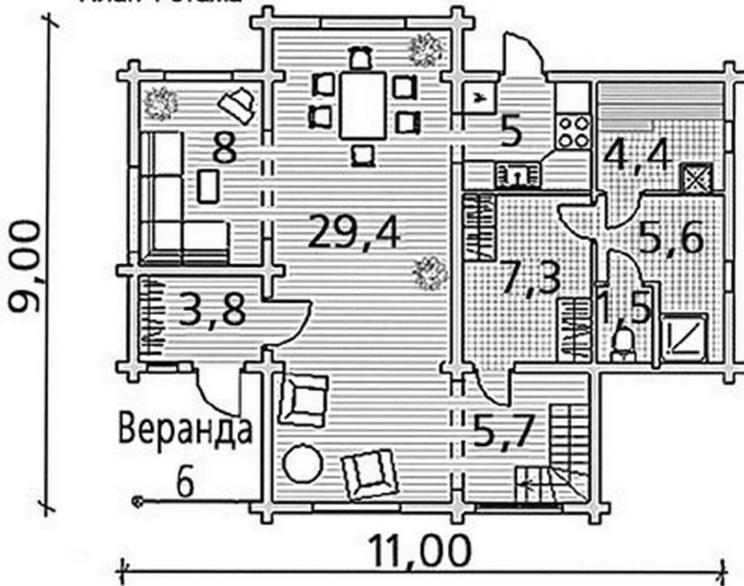
План 1 этажа
