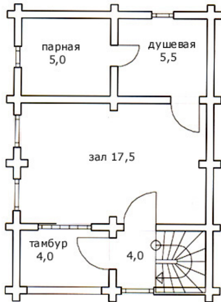
План 1 этажа
