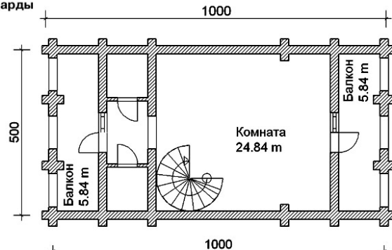
План мансарды
