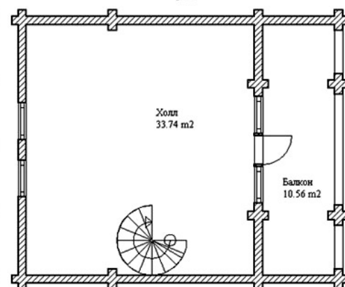
План мансарды
