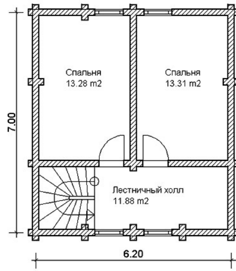
ПЛАН 2-ГО ЭТАЖА
